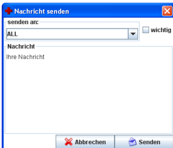
Abb. 1: „Nachricht senden“
