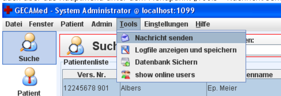
Abb. 1: Menüpunkt „Tools /
